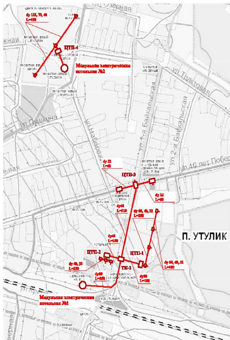
Рисунок 4. Схема теплоснабжения от модульных электростанций № 1, № 2
