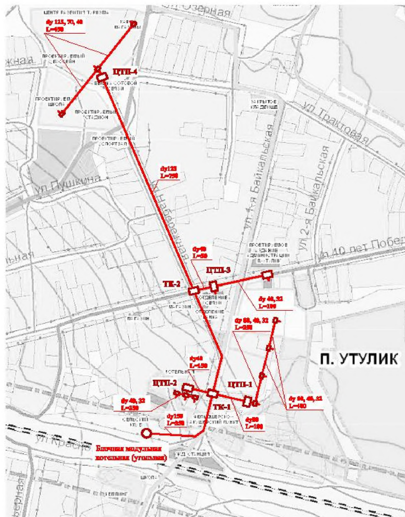
Рисунок 3. Схема теплоснабжения согласно вариант №1.
